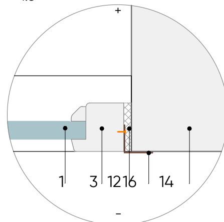
MEZGLS M-104/3
