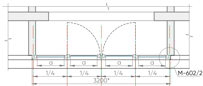
MEZGLS M-602/1
