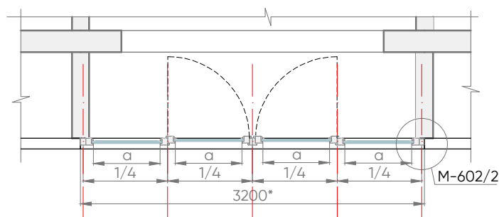
MEZGLS M-602/1
