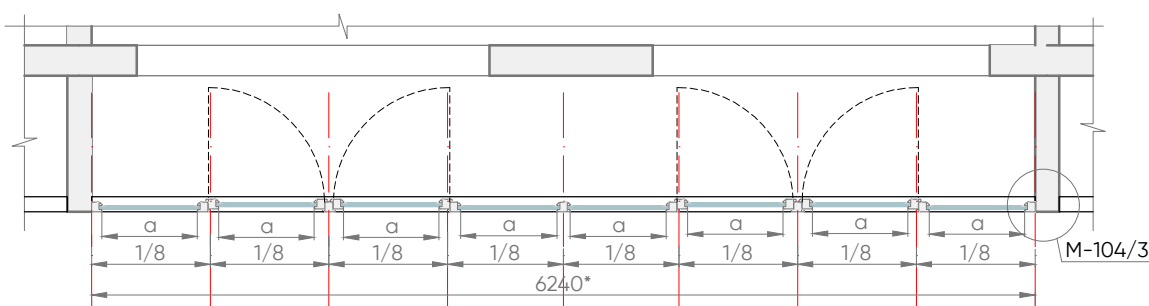
MEZGLS M-104/1
