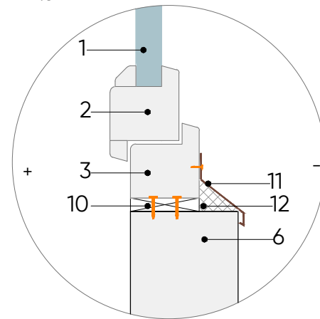
MEZGLS M-103/5
