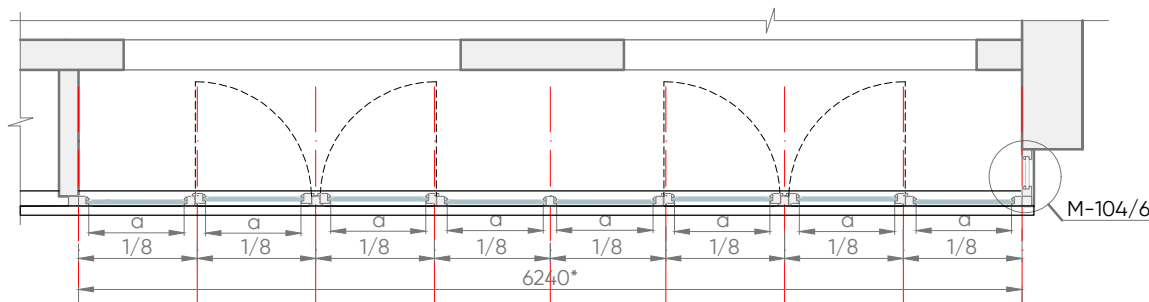
MEZGLS M-104/4
