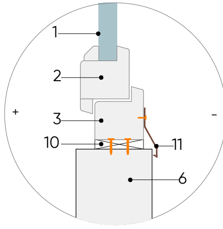
MEZGLS M-119/2
