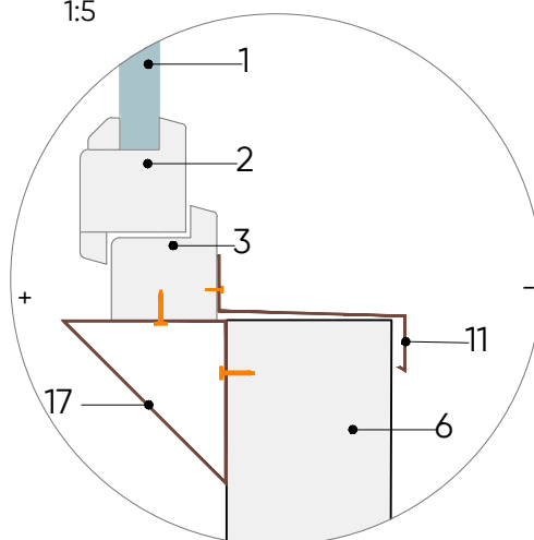
MEZGLS M-103/2 1:5
