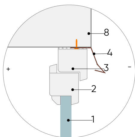
MEZGLS M-119/1
