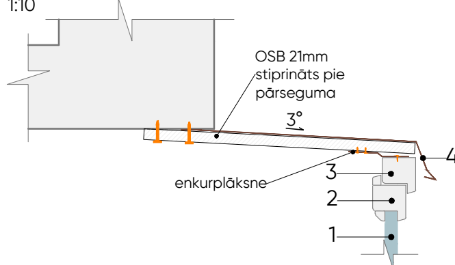
MEZGLS M-119/2
